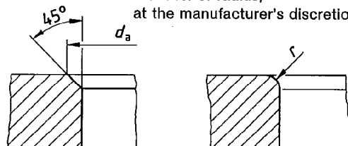
Detail Y
